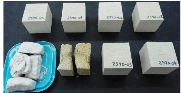
Muestra después de 15 ciclos de ataque de sales Sample after 15 salt attack cycles
